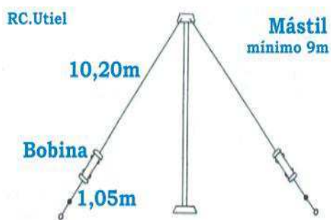
Antena HF DIPOLO MULTIBANDA
